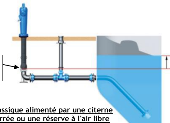
Poteau d'aspiration de 150 mm muni de 2 sorties de 100 mm et d'un carré de manœuvre
